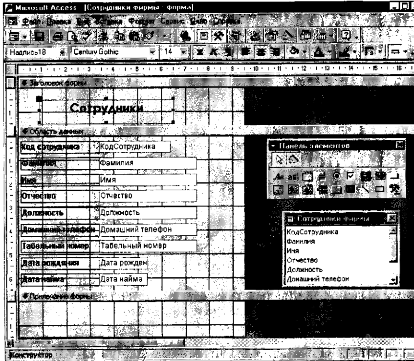
Рис. 18.4. Создание в Конструкторе заголовка формы «Сотрудники»
