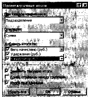
Рис. 10.6. Окно задания параметров расчета промежуточных итогов
